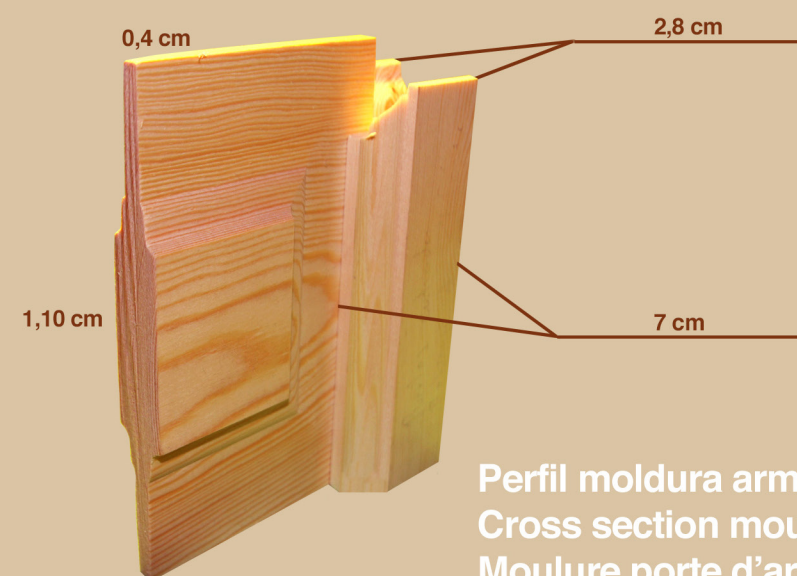
Perfil moldura puerta interior Cross section moulding interior door Moulure porte intérieure
