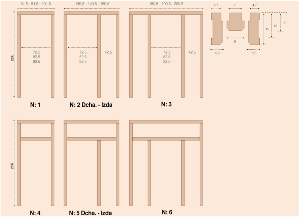
Kits para montar nuestros fabricados en bloque. Kits for block assembly of our manufactured goods Kits pour montage de nos produit en assemblage
